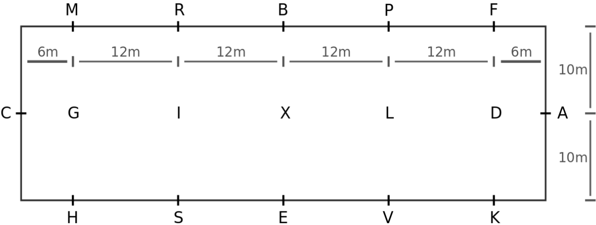
СХЕМА МАНЕЖА 20х60м
